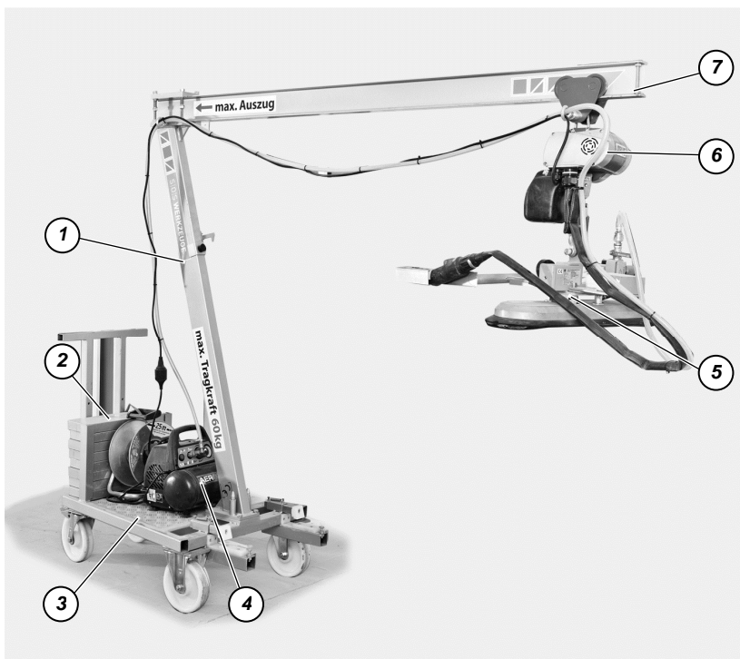
Abb. 1 Fliesenverlegekran Gesamtansicht
